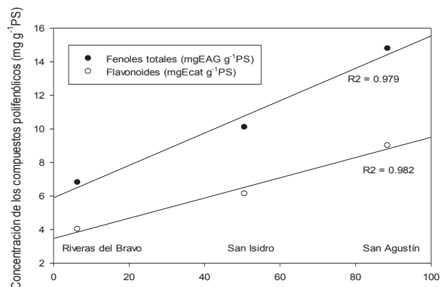
Figura 3. Correlación entre los compuestos fenólicos y nitrato ( \text{NO}_3^- ) disponible en el suelo. EAG -equivalentes a ácido gálico, EC-equivalentes de catequina por gramo ( \text{g}^{-1} ) de peso seco (PS).
