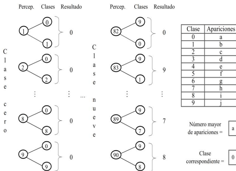
Fig. 3. Red de perceptrones utilizada en el método 1.
