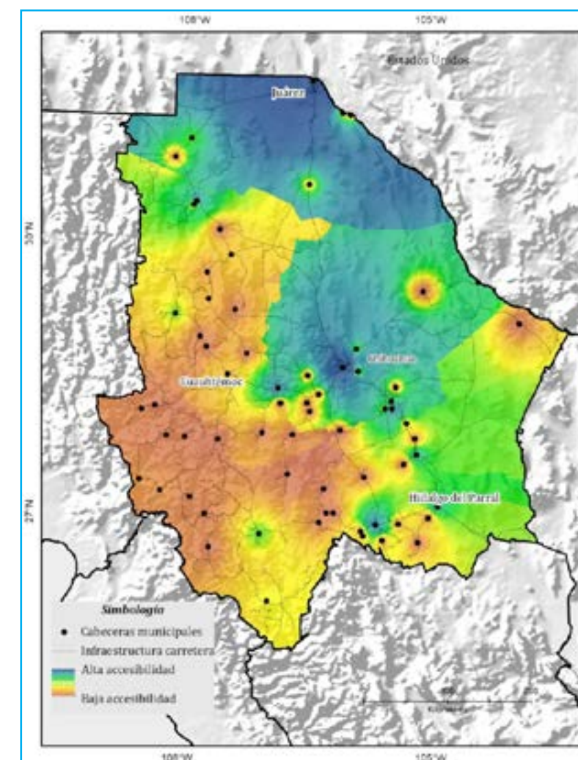
Figura 2. Accesibilidad absoluta de la infraestructura carretera, Chihuahua, México
