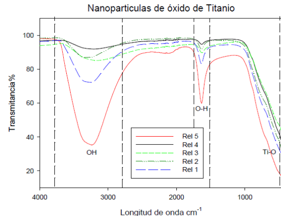
Figura 1. Espectro de infrarrojo de los polvos de \text{TiO}_2 .
