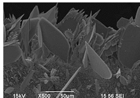
MATERIALES CON FORMA DE PLANTA Hojas de sulfuro de plata que absorben la luz en todo el espectro visible e infrarrojo
