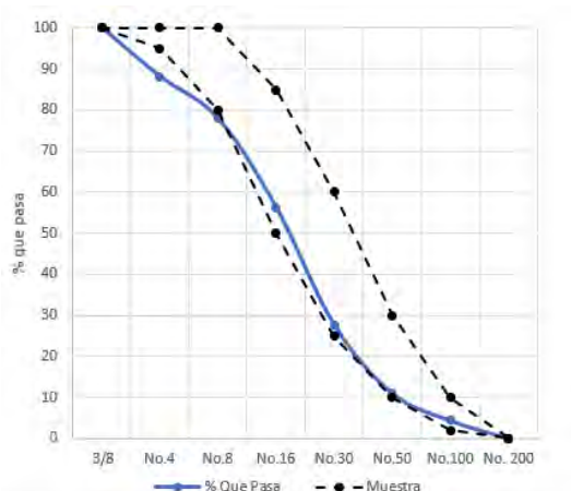
Figura 1. Análisis granulométrico promedio del agregado fino. Fuente: Elaboración propia
