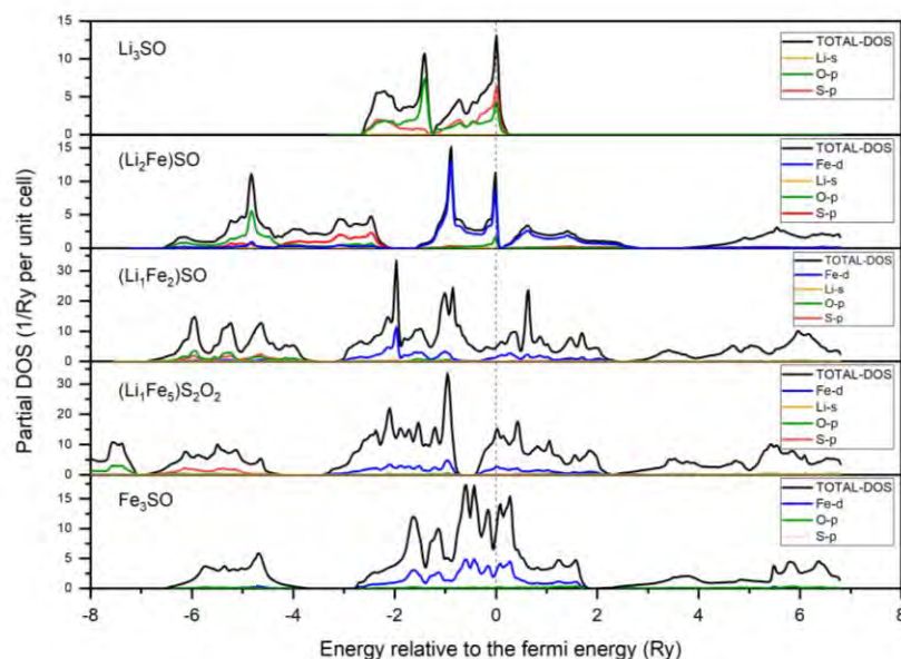
Figura 3. Densidad de los estados total y parciales de la antiperovskita de \text{Li}_3\text{SO} dopado con Fe
