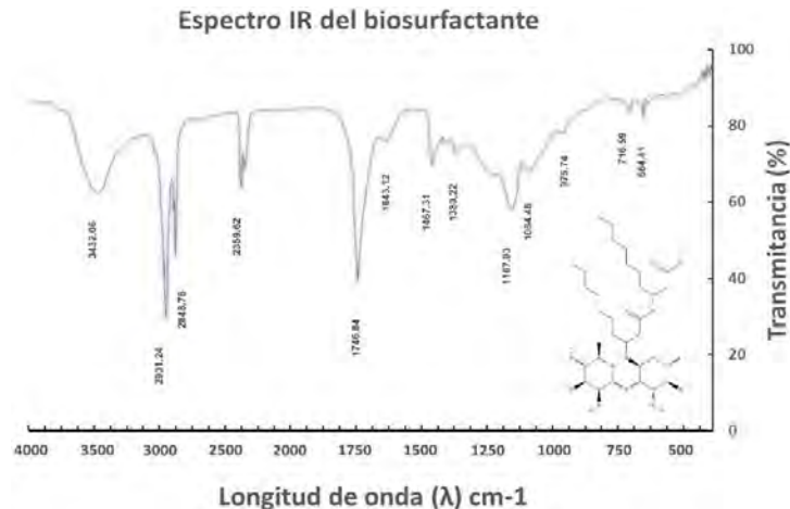
Figura 3. Espectro FTIR del biosurfactante extraído (ramnolípidos).
