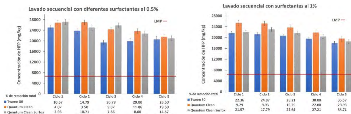
Figura 4. Remoción de HFP con diferentes surfactantes químicos al 0.5% y 1%.
