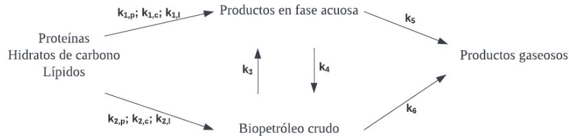
Figura 2. Red de reacción para la licuefacción hidrotérmica de la biomasa microalgal (Valdez et al. , 2014).
