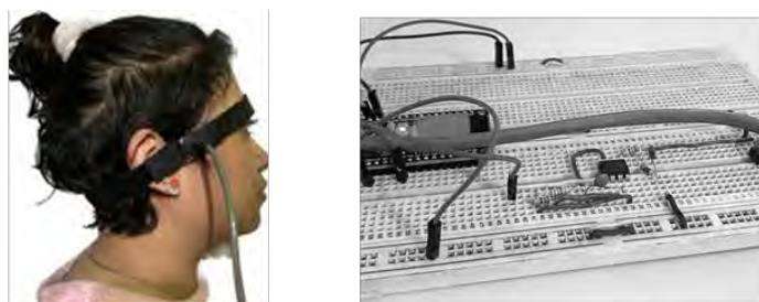
Figura 9. Obtención de la señal mediante fotopletismografía (Fuente: Elaboración propia).
