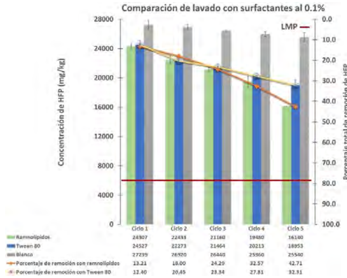
Figura 5. Comparación de lavado con Tween 80 y Ramnolipidos.
