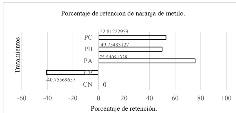
Gráfico 4, Porcentaje de retención de los diferentes carbonos empleados en el ensayo de colorimetría con naranja de metileno, en donde CN: control negativo, CP: control positivo, PA: protocolo A, PB: protocolo B, y PC: protocolo C.
