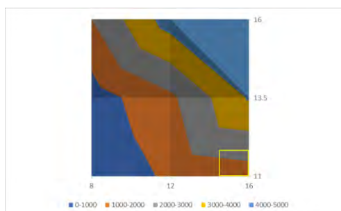
Figura 3: Grafico de contorno de resultados de diseño de experimentos.
