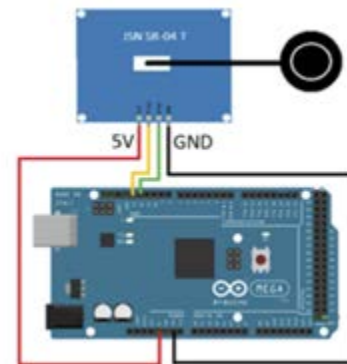
Figura 4. Diagrama eléctrico del sistema con Arduino Mega 2560.
