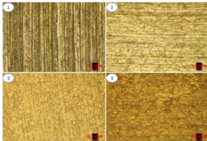
Figura 2. Tipos acabados. Donde: Pieza devastada 1) Acabado de lija grado 60, 2) Acabado de lija grado 320, 3) Acabado de lija grado 800, 4) Acabado de lija grado 1200.
