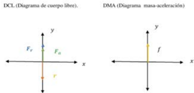
Figura 3. Diagramas de cuerpo libre y de masa-aceleración.
