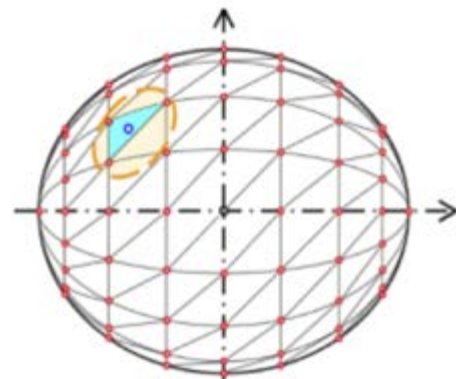
Figura 3. Modelación del grano. Fuente: Elaboración propia.
