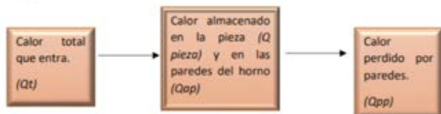
Figura 1. Balance de energía. Fuente: Elaboración propia.
