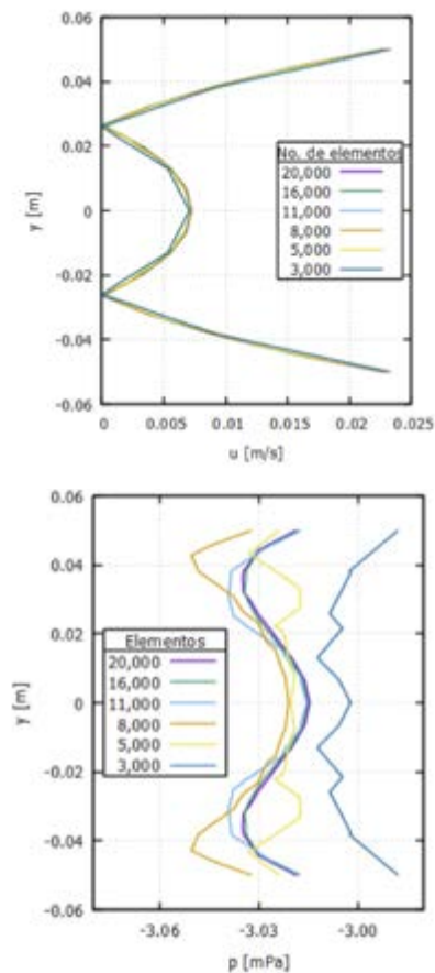
Figura 9. Perfil de velocidad y presión para dominio rectangular. Fuente: Elaboración propia.
