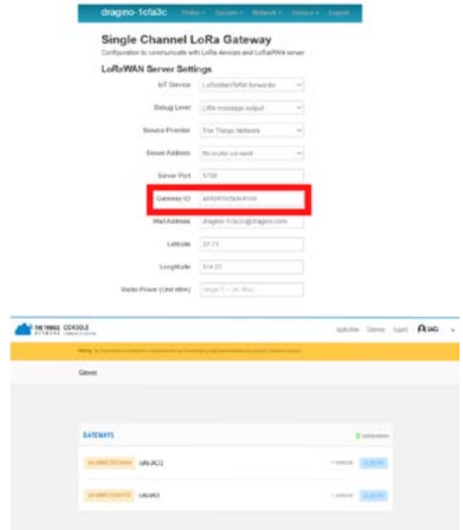
Figura 8. Conexión del Gateway al Servidor. Fuente: Elaboración propia.
