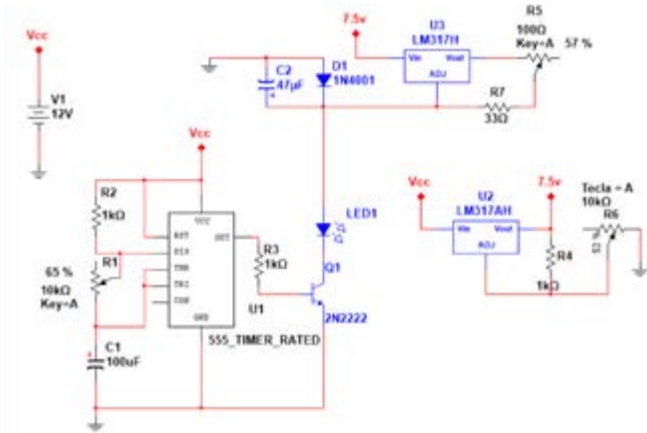
Figura 5. Control para láser terminado. Fuente: Elaboración Propia.
