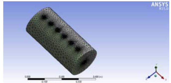
Figura 4. Malla tridimensional en un conducto de 0.040m de diámetro con refinamiento en la zona del grano. Fuente: Elaboración propia.
