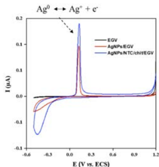
Figura 2. Voltamperometría cíclica sobre EGV pulido (línea negra), EGV modificado con nano-partículas de plata (línea roja) y EGV modificado con NTCPM/Chit/NpAg en solución de HCl\ 0.1M a 0.05\ Vs^{-1}
