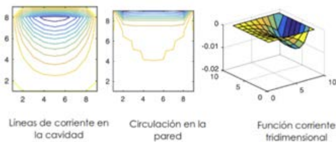
Figura 10. Respuesta a velocidad de 0.3133 m/s. Fuente: Elaboración propia.
