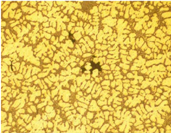
Figura 3. Pieza con pulido acabado espejo en paño con sílica coloidal. Fuente: Elaboración Propia.
