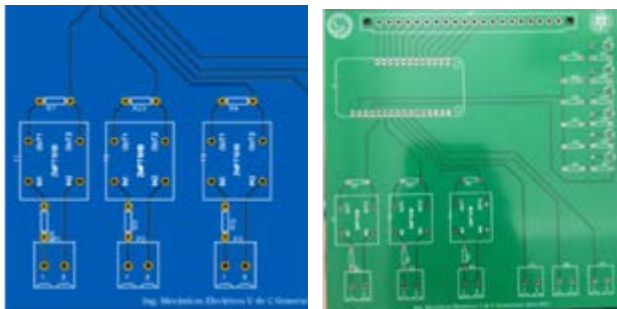
Figura 4. Diseño de la PCB en EasyEDA.com (arriba) y en físico (abajo). Fuente: Elaboración propia.
