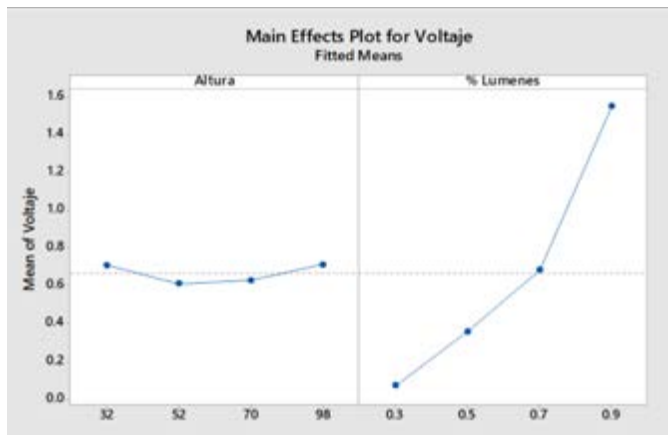
Figura 10. Gráfica de Efecto Principales Altura- Voltaje.
