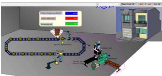
Figura 7. Modelo de simulación del proceso. Fuente: Elaboración propia.
