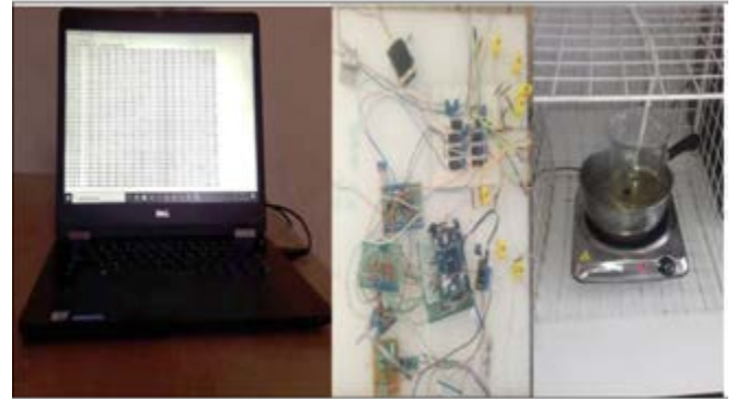
Figura 3. Interconexión Hardware y Software. Fuente: Elaboración propia.
