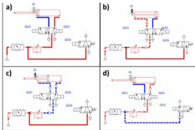
Figura 8. Etapas del proceso neumático.
