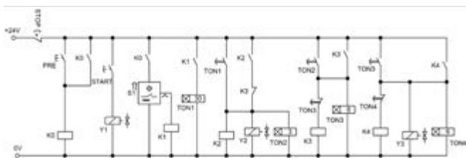
Figura 6. Diagrama del sistema de control. Fuente: Elaboración propia.
