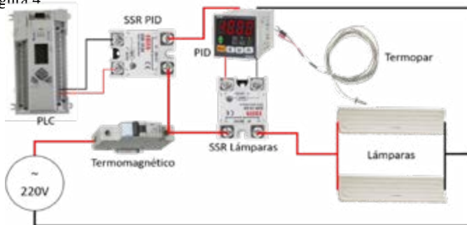
Figura 4. Esquema eléctrico para las lámparas de radiación infrarroja. Fuente: Elaboración propia.
