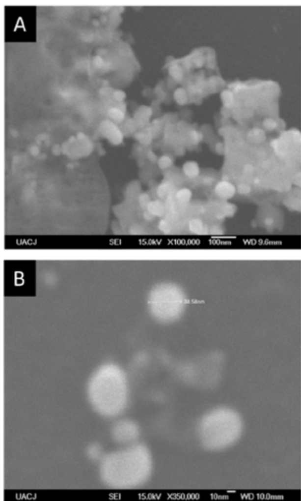
Figura 3. Imágenes de SEM de la superficie de electrodo EGV, modificada con AgNp: a) 100,000X, y b) 350,000X. Fuente: Elaboración propia.
