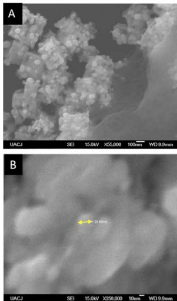
Figura 4. Imágenes de SEM de la superficie de electrodo EGV/NTCPM/Chit/ con AgNp: a) 55,000X SEI y b) 350,000X. Fuente: Elaboración propia.
