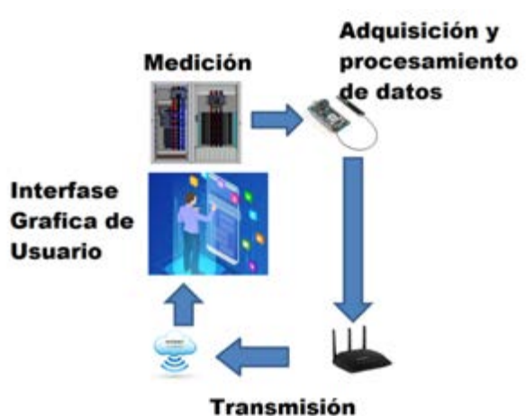
Figura 1. Diseño general del sistema. Fuente: Elaboración propia.
