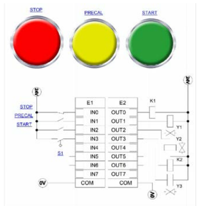
Figura 7. Conexiones de entrada y salida del PLC. Fuente: Elaboración propia.
