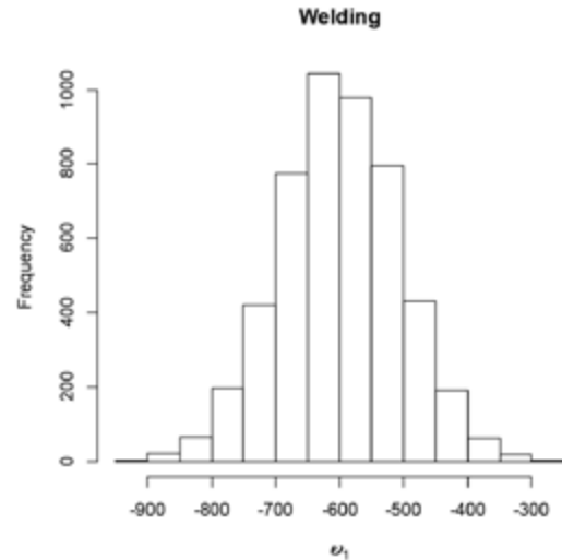
Figura 6. Predicción del comportamiento del coeficiente del tiempo de soldadura. Fuente: Elaboración propia.
