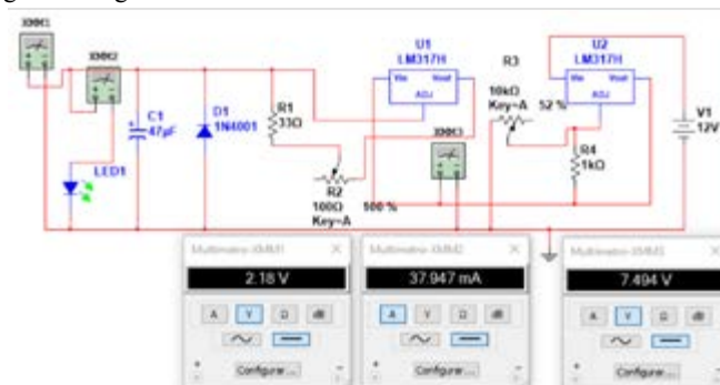
Figura 4. Diseño de fuente de corriente de 0.01 a 0.250 A. Fuente: Elaboración Propia.
