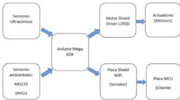
Figura 1. Esquema del sistema solución. Fuente: Elaboración propia.
