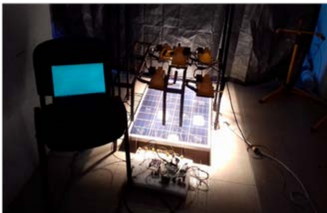
Figura 4. Arreglo de Lámparas y Celda Para Obtención de Datos.
