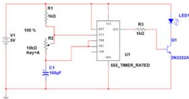
Figura 3. Circuito astable con circuito integrado NE555. Fuente: Elaboración Propia.
