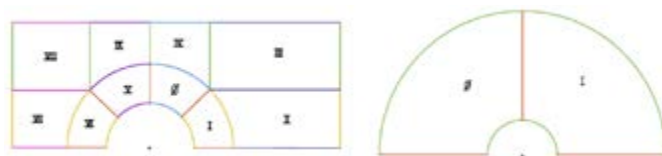
Figura 2. Bloques para el mallado de cada dominio geométrico.
