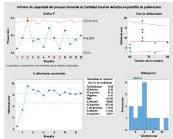
Figura 6. Análisis de capacidad del proceso binomial. Fuente: Elaboración propia.
