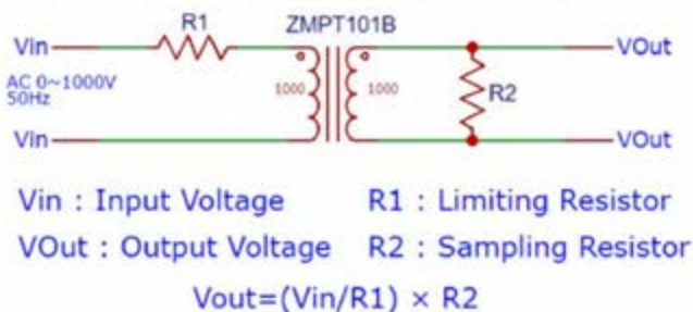
Figura 2b. Circuito equivalente del sensor ZMPT101B. Fuente: Elaboración propia.
