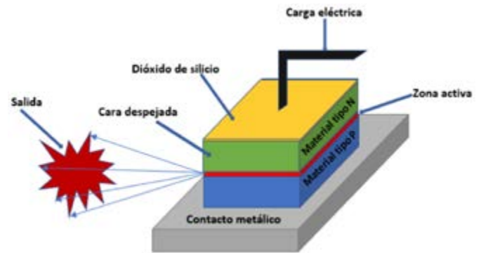
Figura 2. Esquema de un láser semiconductor.
