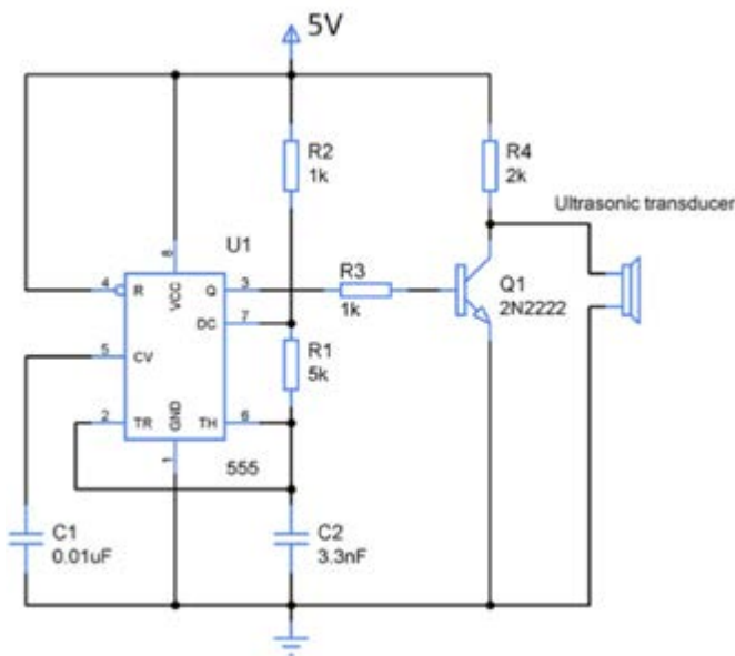
Figura 9. Sistema con LM555.
