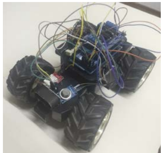
Figura 4. Vista del rover propuesto. Fuente: Elaboración propia.
