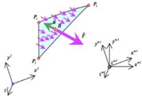
Figura 9. Presión y fuerza resultantes superficial sobre el grano. Fuente: Elaboración propia.
