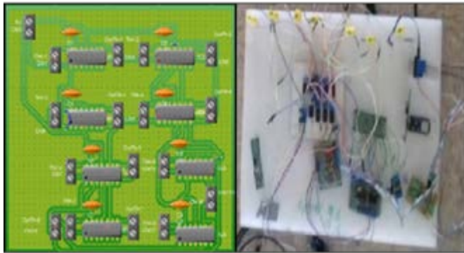
Figura 1. Tarjeta de Adquisición de Datos. Fuente: Elaboración propia.
