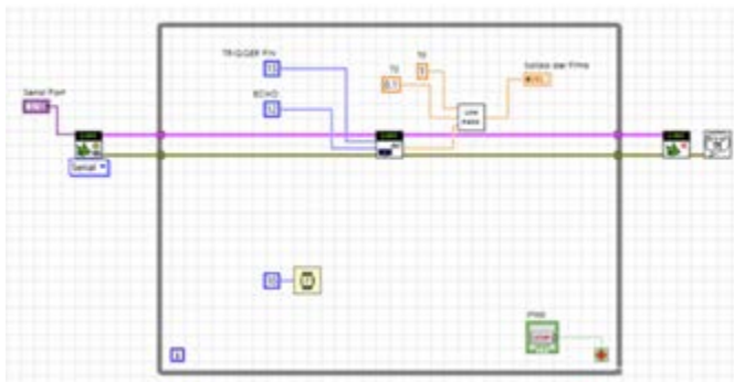
Figura 2. Diagrama a bloques del sistema. Fuente: Elaboración propia.
