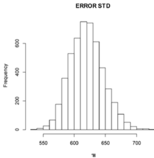
Figura 8. Comportamiento del Error Estándar. Fuente: Elaboración propia.
