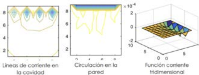
Figura 12. Respuesta a velocidad de 0.3133 m/s. Fuente: Elaboración propia.
