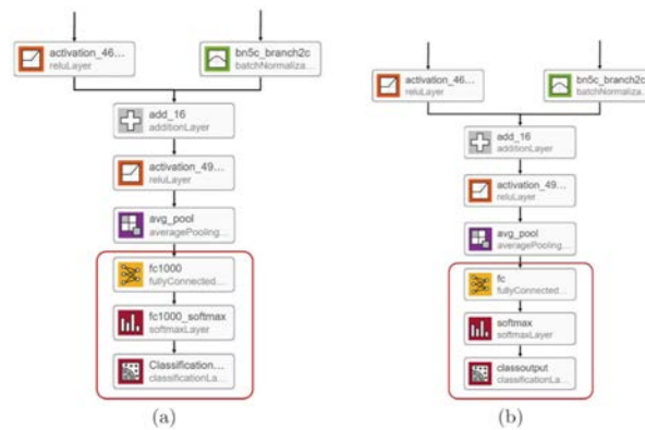
Fig. 6. Cambios realizados a la red ResNet-50. (a) Capas finales originales de ResNet-50, (b) Capas finales modificadas a ResNet-50.
