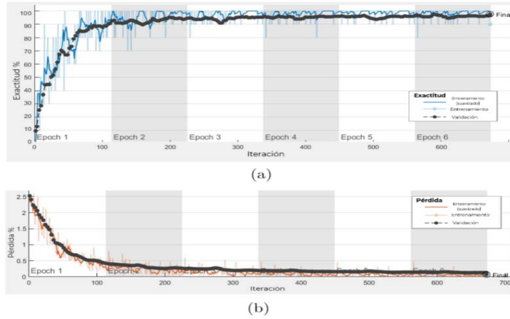
Fig. 7. Gráfica de (a) exactitud y (b) pérdida en el entrenamiento de la CNN.
