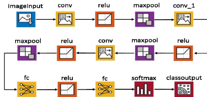
Fig. 5. Arquitectura de CNN para entrenamiento con CIFAR-10.
