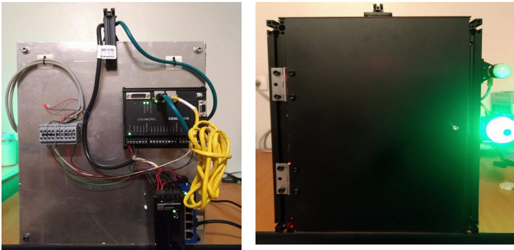
Figura 11. Vistas del sistema de visión montado en la máquina clasificadora
