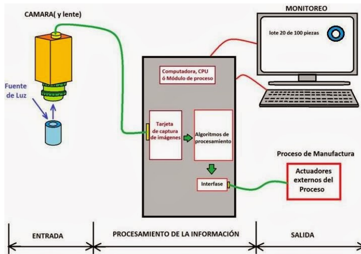
Figura 1. Etapas de un sistema de visión.
