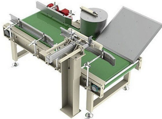
Figura 5. Vistas del clasificador empleado en el proyecto.
