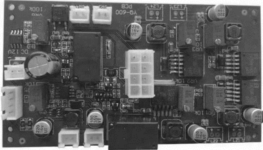
Figura 7. Pieza patrón para el algoritmo de visión.
