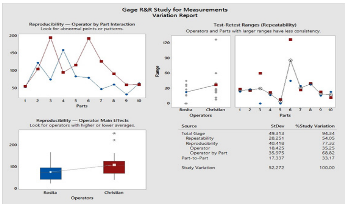
Figura 4. Resultado de estudio R&R del sistema de medición mejorado para tamaño de partículas.
