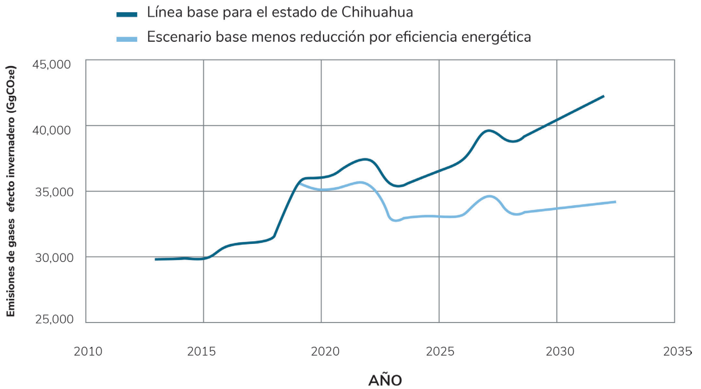
Figura 20. Comparativo del escenario base de emisiones de gases de efecto invernadero en CO 2 e con el escenario en el que se aplican medidas de eficiencia energética exclusivamente.
