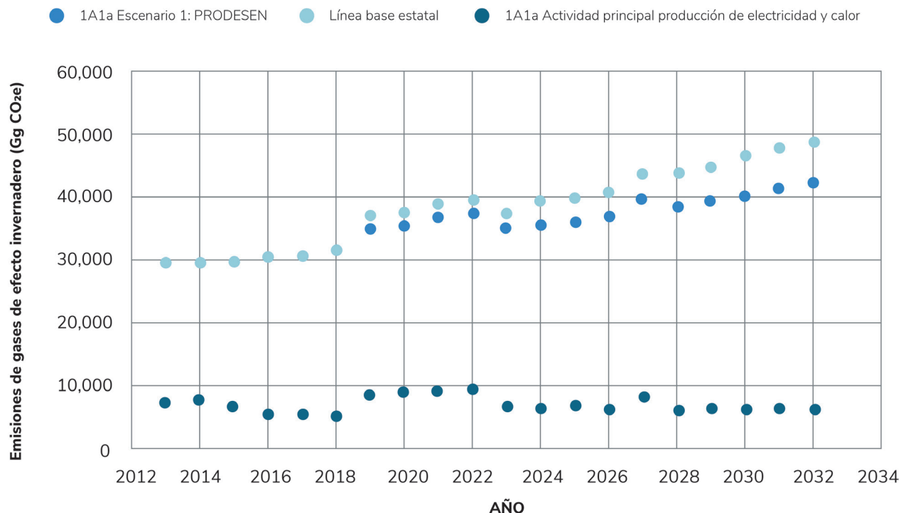
Figura 17. Efecto de las medidas de mitigación a la ampliación de la capacidad de generación eléctrica del estado de Chihuahua.
