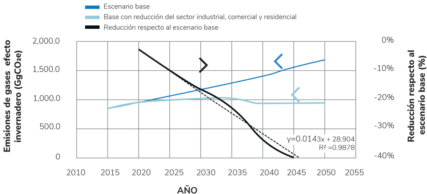
Figura 19. Efecto de las medidas de eficiencia energética en los sectores económicos industrial, comercial y residencial.
