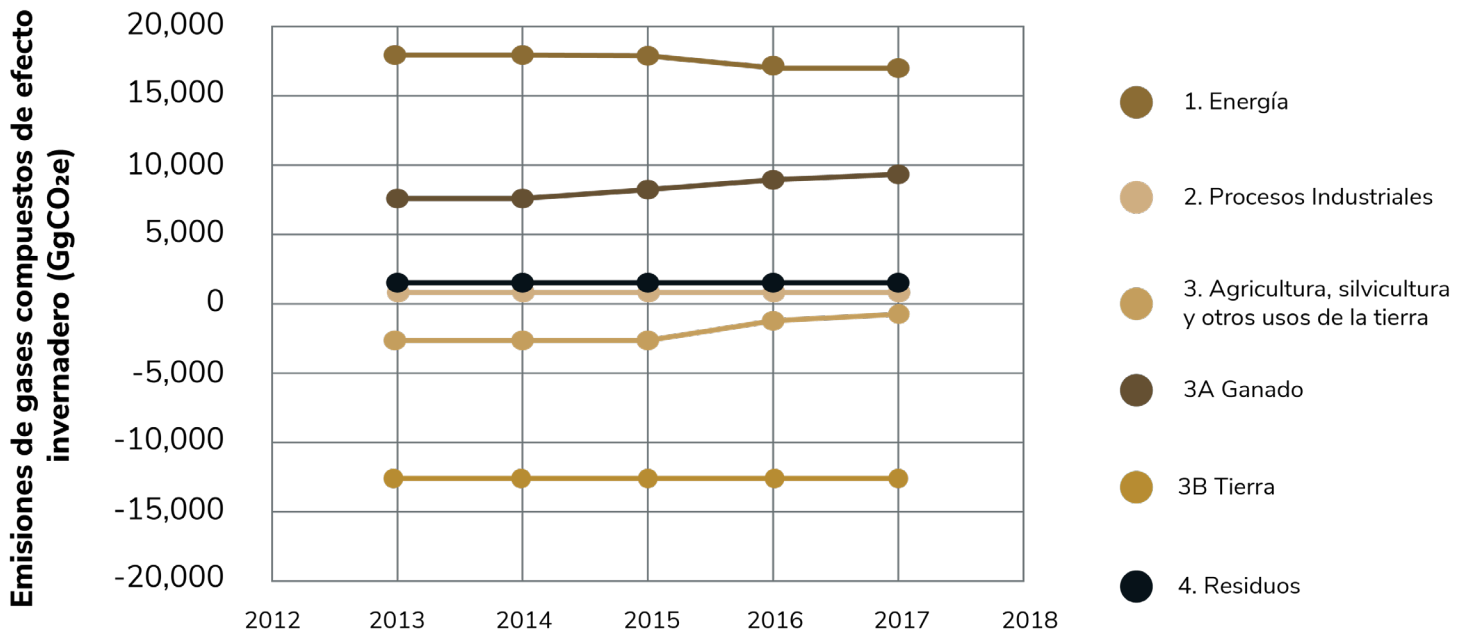
Figura 11. Inventario de emisiones de gases de efecto invernadero.
