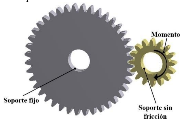
Figura 3. Aplicación de rotación y momento.
