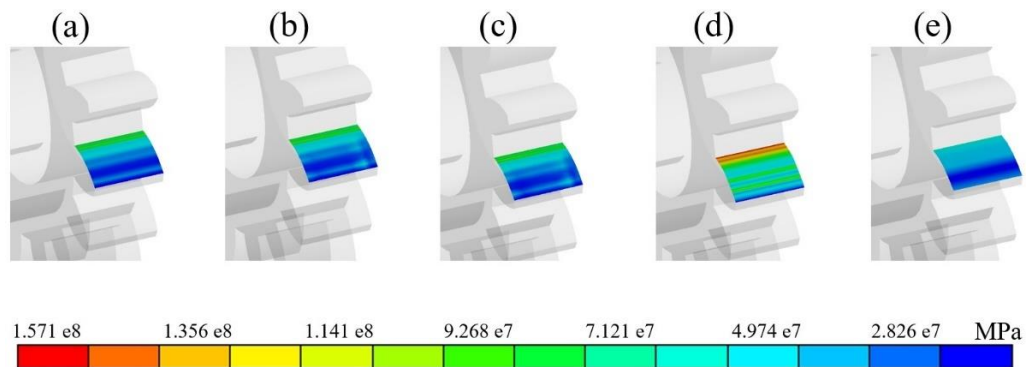
Figura 6. Esfuerzos alternantes en diente del engrane piñón, a) base, b) axial M0.2, c) axial M0.3, d) radial M0.2, e) radial M0.5
