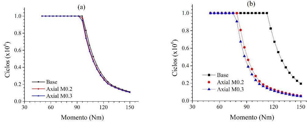
Figura 5. Ciclos de vida con desalineamiento axial, a) diente de engrane piñón, b) diente de engrane rueda
